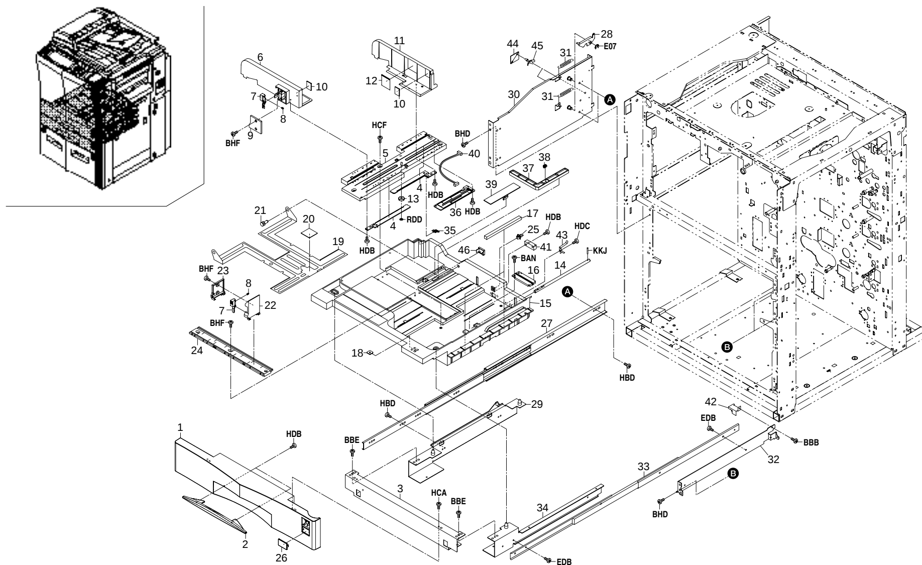
FIG. 3 CASSETTE SECTION
